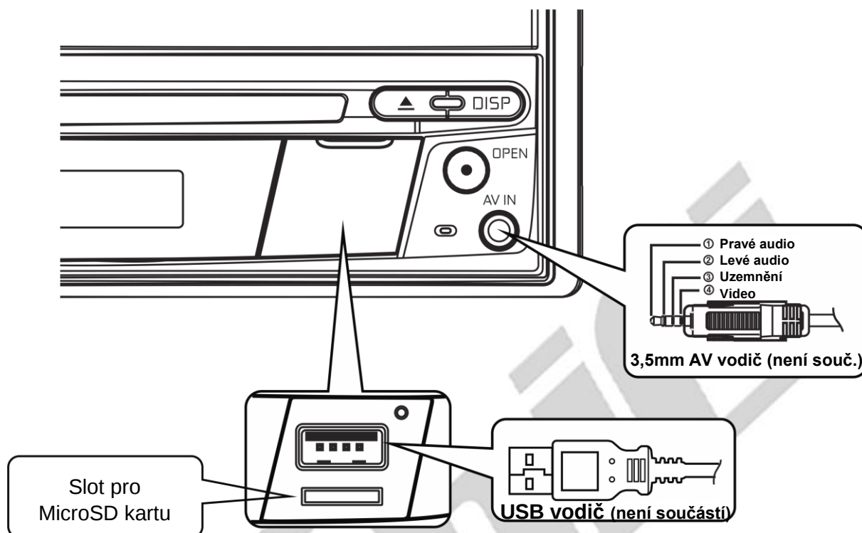
MAC 410 Umístění USB slotu a slotu pro MicroSD kartu
